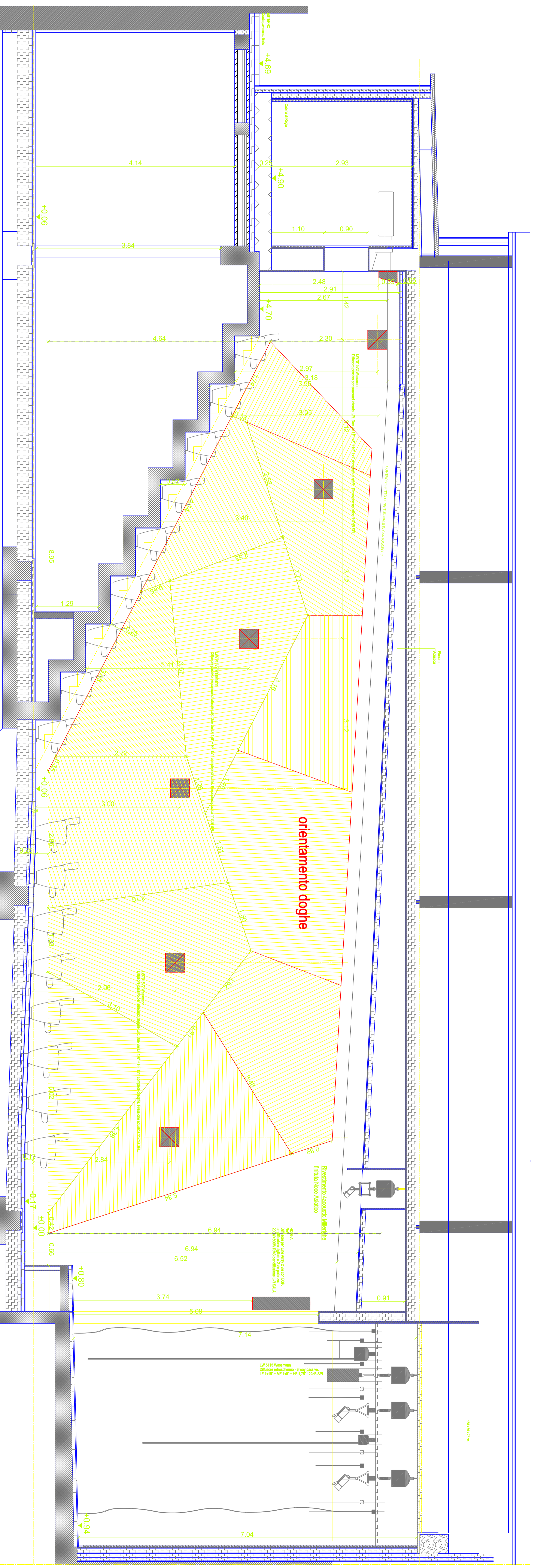
PROSPETTO LATO B SEZIONE CENTRO SALA CINEMATOGRAFO - Scala 1.50 Posizionamento pannelli Fantoni
